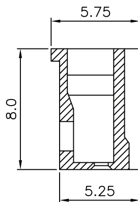
A-A SEC
