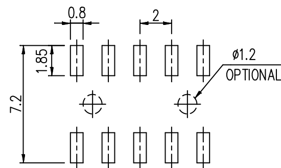
P.C.B. LAYOUT
